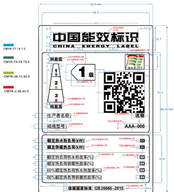
图3 燃气采暖热水炉(两用型)能源效率标识样式示例
