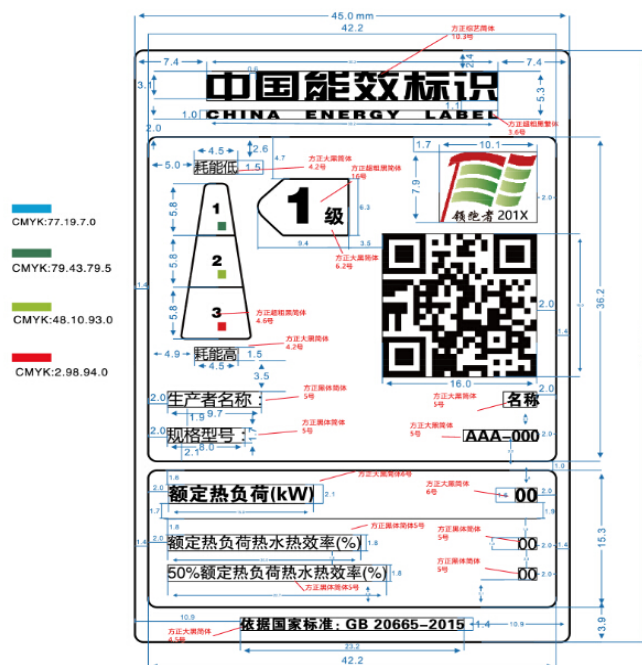
图 1 家用燃气快速热水器能源效率标识样式示例
