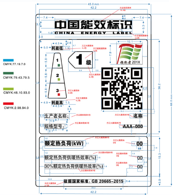
图 2 燃气采暖热水炉（单采暖型）能源效率标识样式示例
